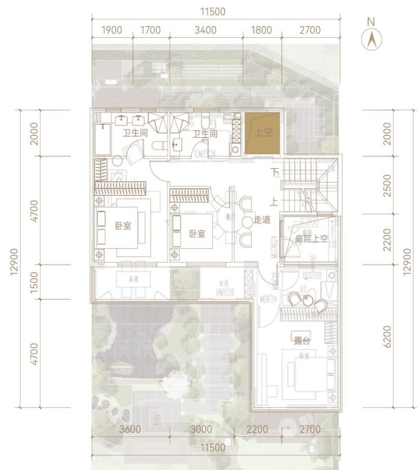
二层平面布置图 (改造后) FLOOR PLAN
